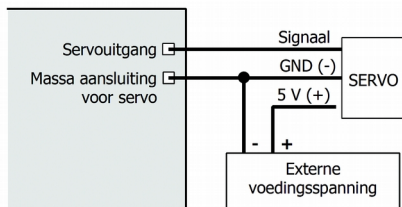
Fig. 5: Aansluiten van een servo
