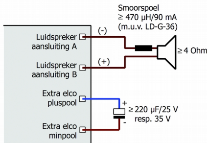
Fig. 4: aansluiten van een elco voor het verbeteren van de voeding en een smoorspoel op de luidspreker.
