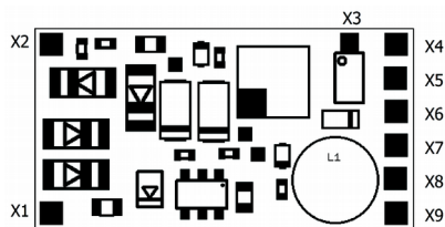
Fig. 1: Aansluitingen
