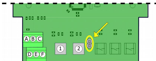
letztes Gleismodul
