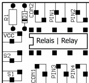
Fig. 1: Bestückungsplan
