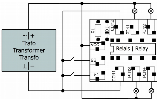
Fig. 2: Plan de connexion
