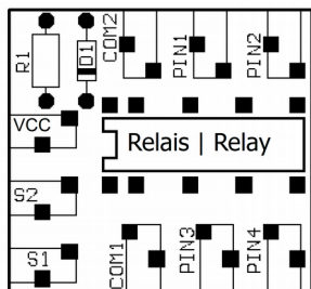
Fig. 1: Plan d'implantation
