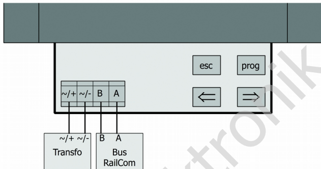
Fig.1: Connexions du RCA-24
